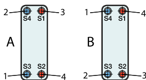
Figura 5. Circuito simple: A evaporador; B condensador.
